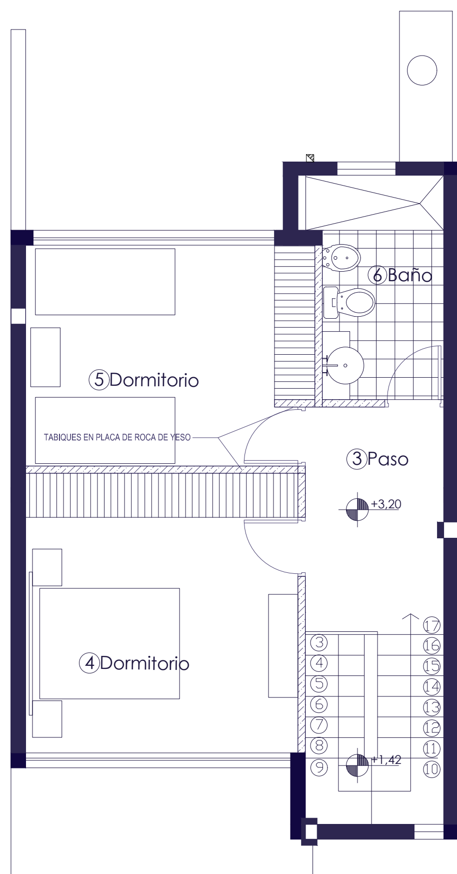
Planta alta
