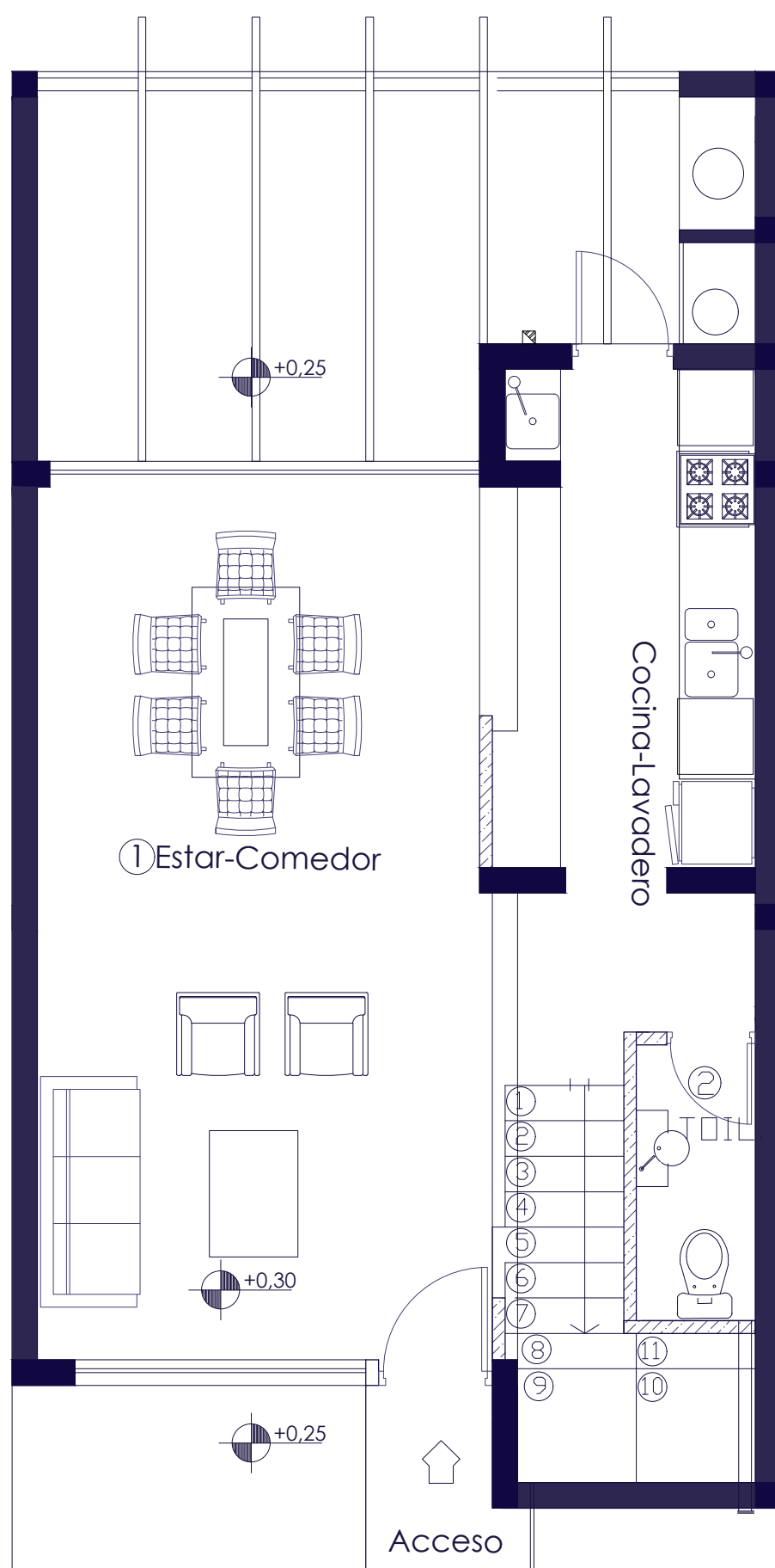
Planta baja
